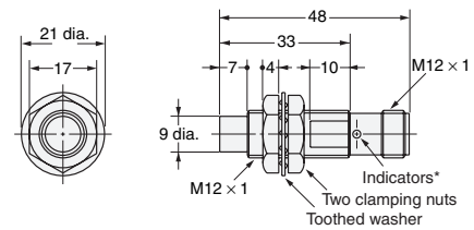
Diagram 21 E2E-X8MD□-M1(G) E2E-X5ME□-M1/E2E-X5MF□-M1
