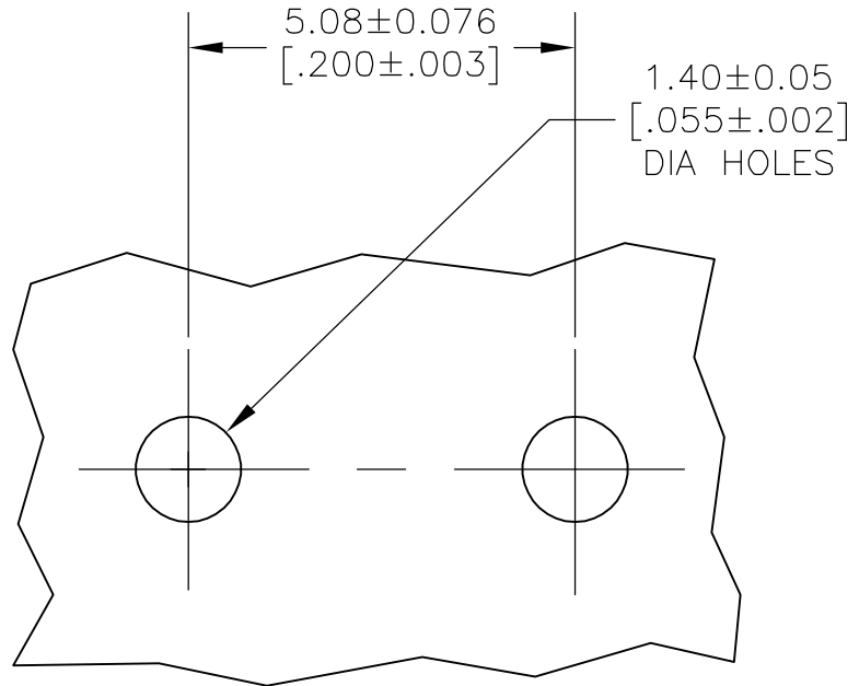
P.C.BOARD HOLES
