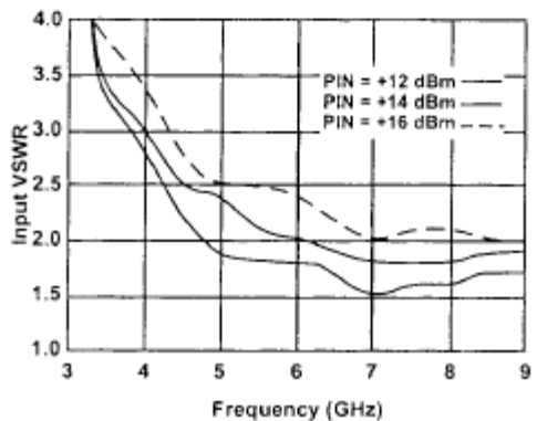
Input VSWR
