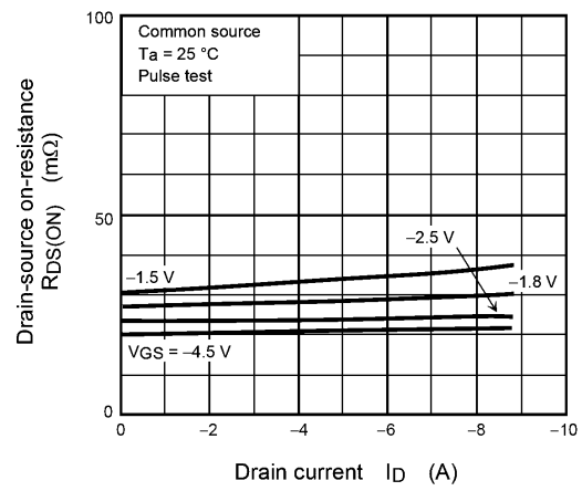
Fig. 7.4 R_{DS(ON)} - I_D
