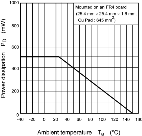
Fig. 7.13 P_D - T_a
