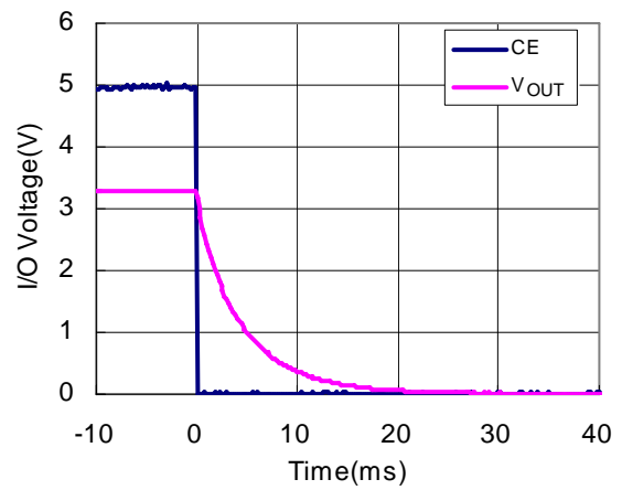
RP501K331A
