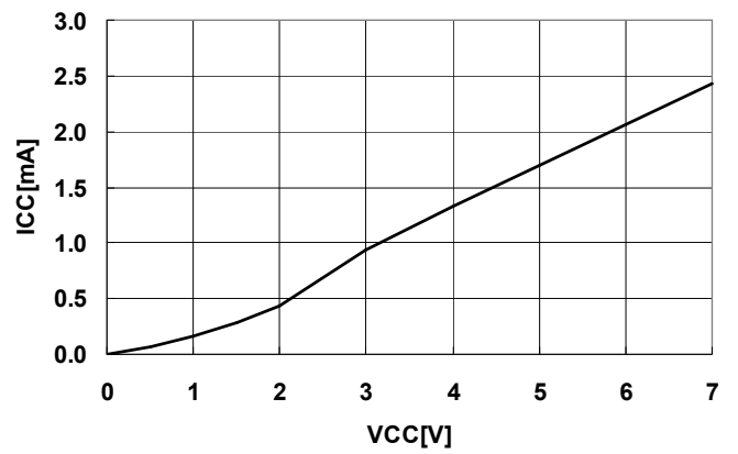
VDD VS. IDD2 INPUT=L T_a=25[^\circ\text{C}]
