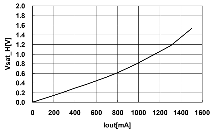
Iout VS. Vout VDD=7V T_a=25[^\circ\text{C}]
