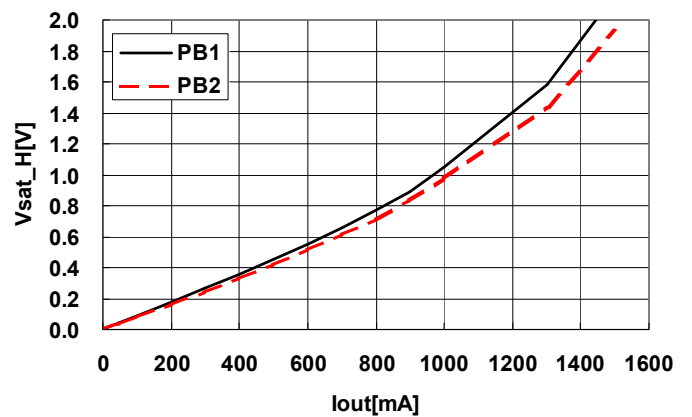
Iout VS. Vout VDD=5V T_a=25[^\circ\text{C}]
