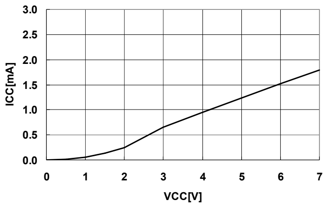
VDD VS. IDD1 INPUT=H T_a=25[^\circ\text{C}]
