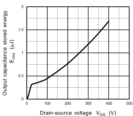
Fig. 8.10 E_{OSS} - V_{DS}
