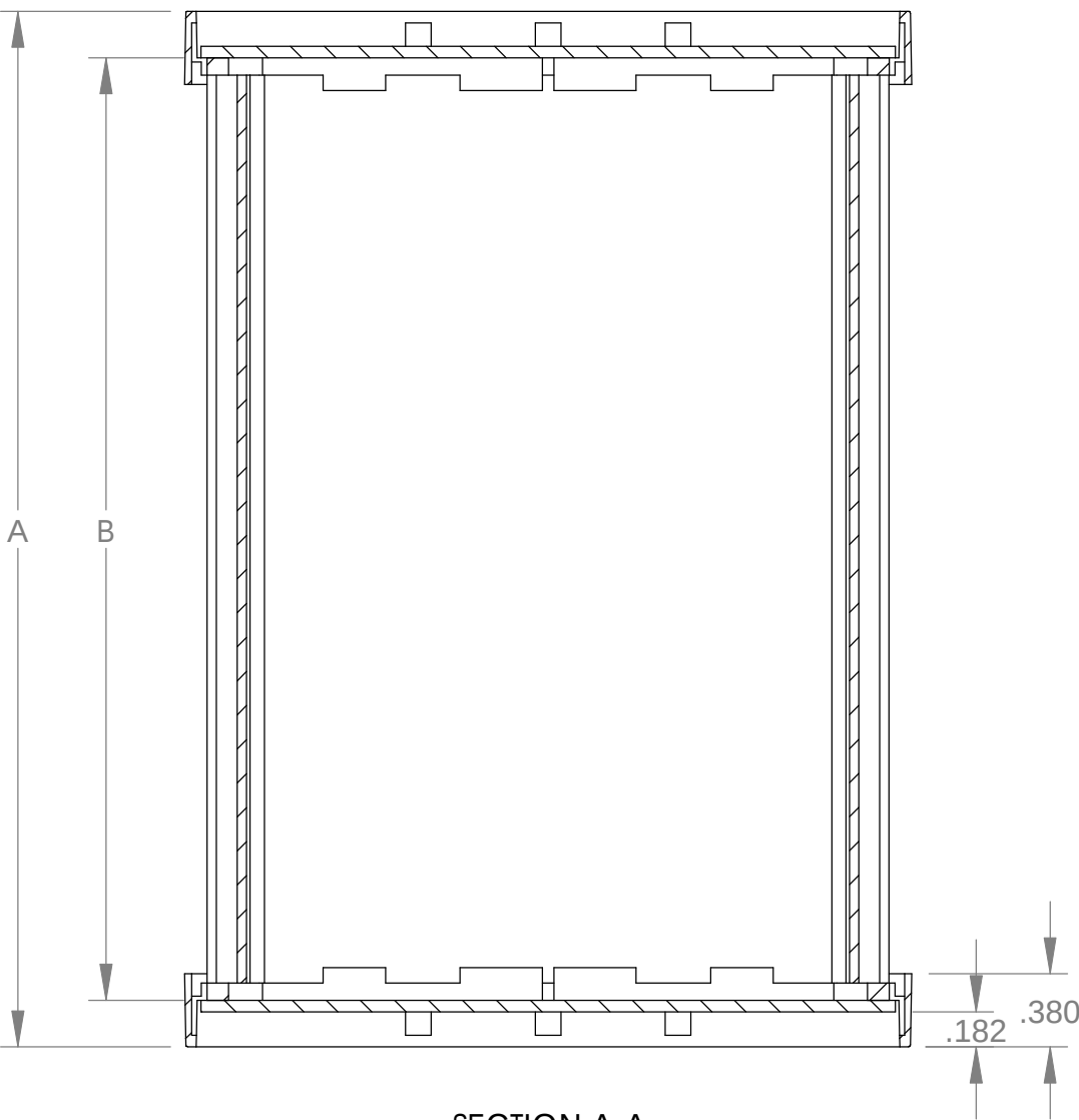
SECTION A-A
