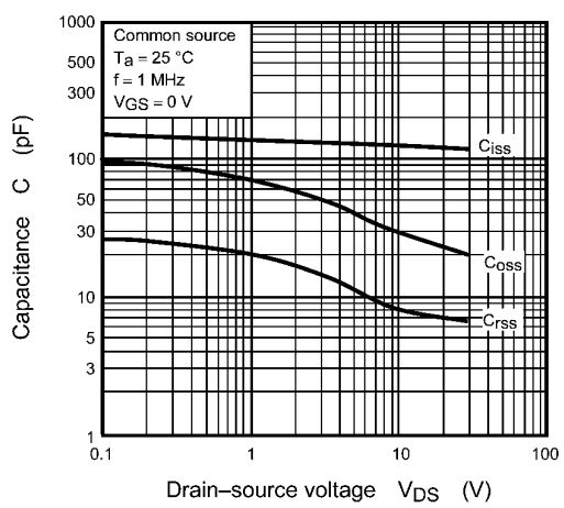
Fig. 7.10 C - V_{DS}
