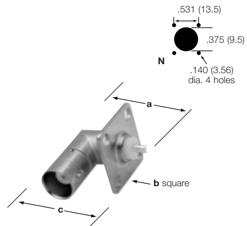
BNC Angle Panel Receptacle 5675
