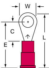
MVU18-10R/L Stud Size 10 Wire Range 22-18
