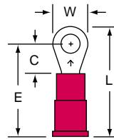
MVU18-6R/S Stud Size 6 Wire Range 22-18
