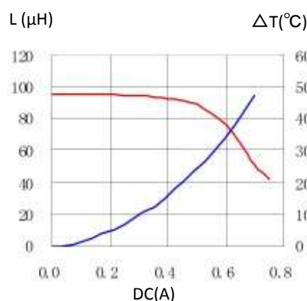
9. CDRR73NP-101MC
