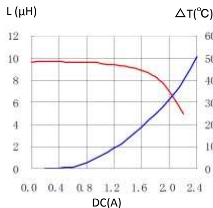
3. CDRR73NP-100MC
