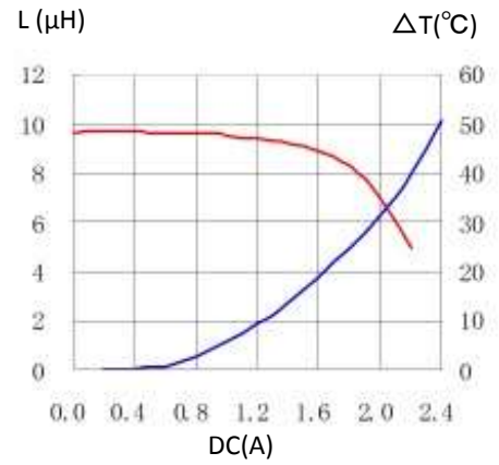
3. CDRR73NP-100MC
