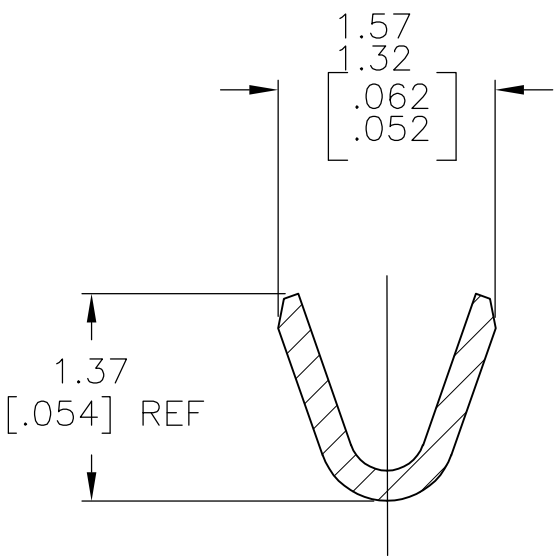
SECTION A-A SCALE 20:1
