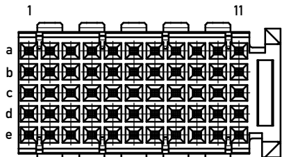
Bestückungsplan / contact layout
