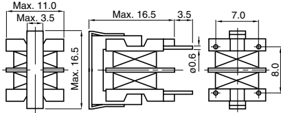
DIMENSIONS (mm) 外形寸法図
