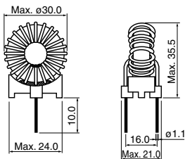
DIMENSIONS (mm) 外形寸法図
