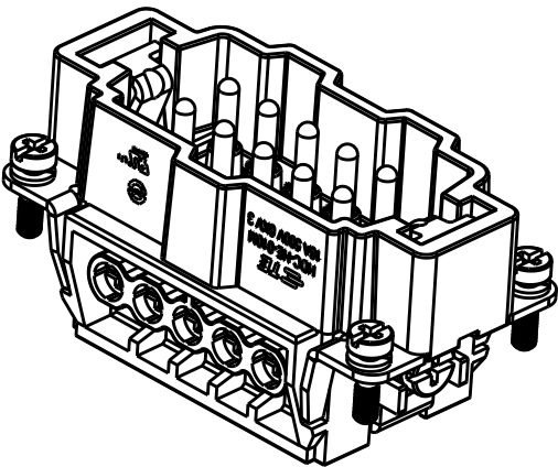
TYPE 1, T2040102101-000, WITH LOGO 类型 1, T2040102101-000, 带LOGO
