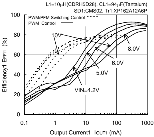
FOSC=500kHz, VOUT1=3.3V
