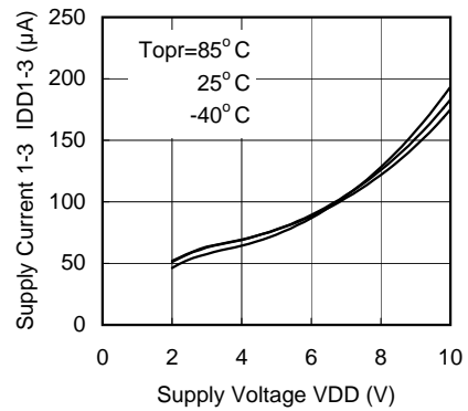
XC9505B095 (180KHz)
