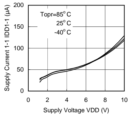
XC9505B092 (180KHz)
