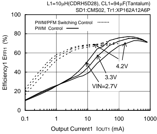
FOSC=500kHz, VOUT1=1.0V
