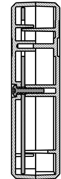
SECTION D-D
