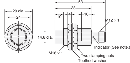
Fig. 24 : E2E-X14MD□-M1(G)/E2E-X10ME□-M1/F□-M1 E2E-X10MY□-M1
