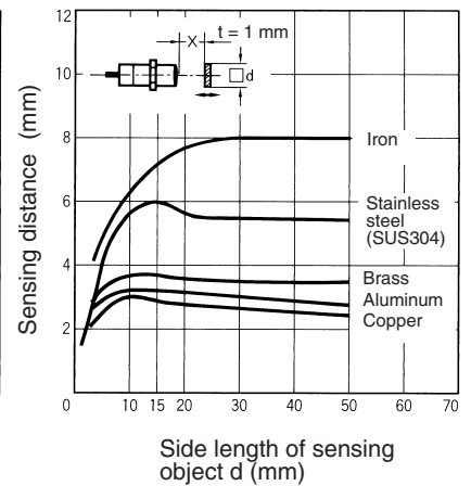
E2E-X1R5E/F E2E-X1R5Y
