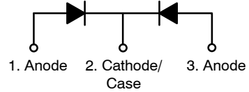
Schottky Diode
