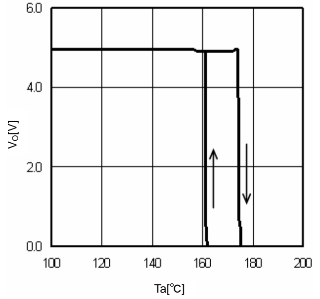
Fig.16 TSD ( I_o=0\text{mA} )
