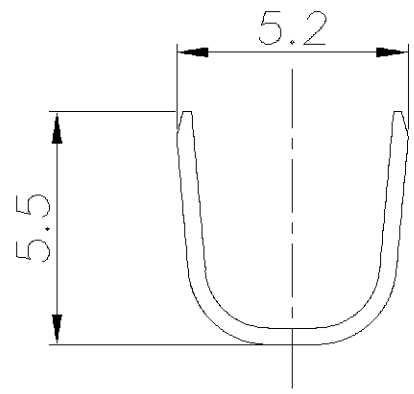
SEC. A-A
