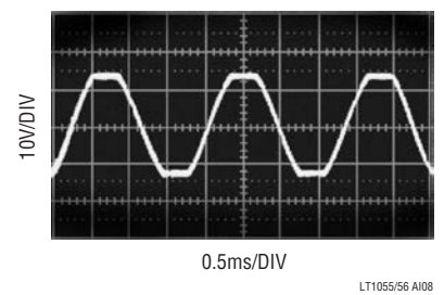
Output LT1055/LT1056
