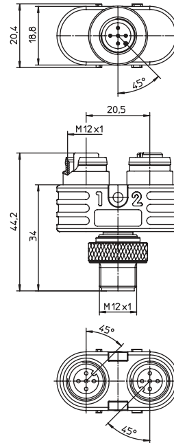
FASBS 2 M12
