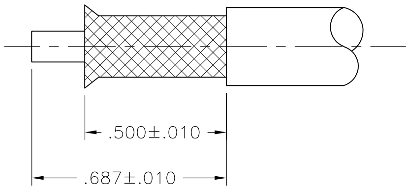
DETAIL Y
