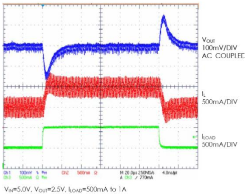
Fig. 20: Load Step
