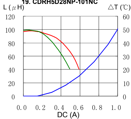
19. CDRH5D28NP-101NC
