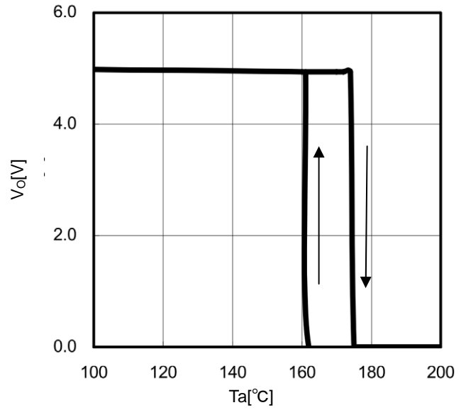
Figure 28. TSD ( I_o=0\text{mA} )
