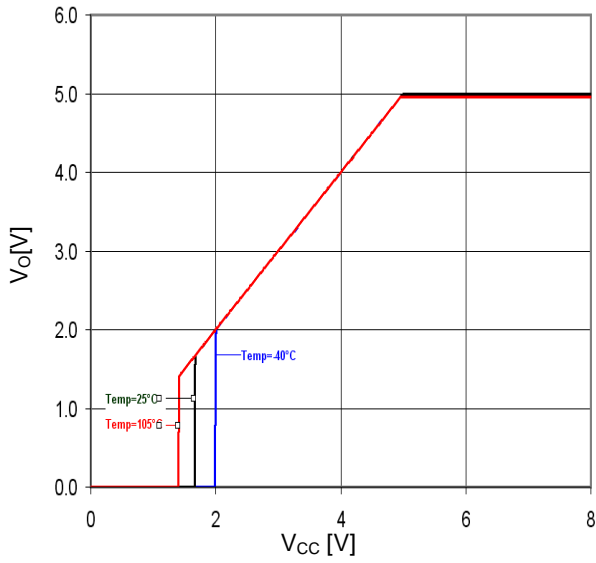
Figure 27. Vcc-Vo ( I_o=0\text{mA} )
