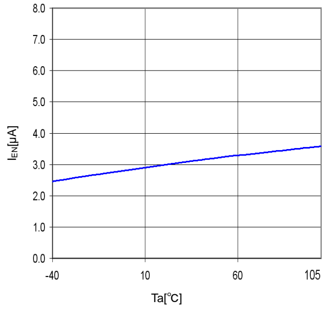
Figure 24. Ta-I EN
