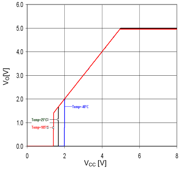
Figure 27. Vcc-Vo ( I_o=0\text{mA} )
