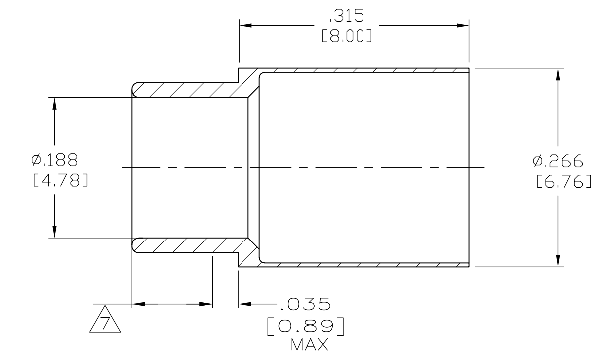
1 4 FERRULE
