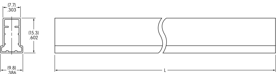
Stick-Tube Dimensions
