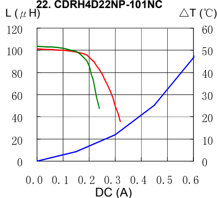
22. CDRH4D22NP-101NC
