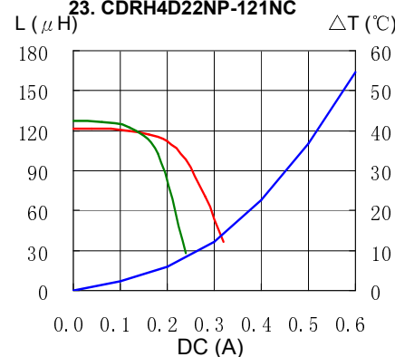
23. CDRH4D22NP-121NC
