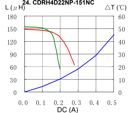
24. CDRH4D22NP-151NC
