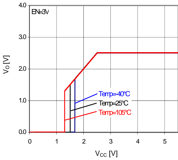
Fig.27 V_{cc}-V_o ( I_o=0mA )
