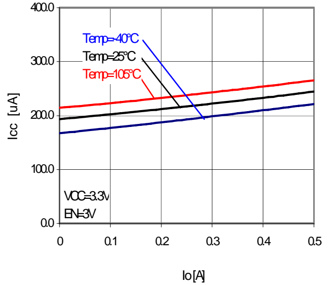
Fig.30 I_o-I_{cc}
