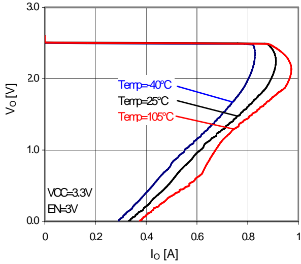
Fig.29 OCP
