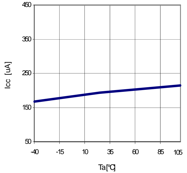
Fig.22 Ta-I cc
