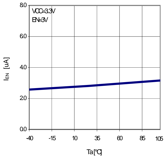
Fig.24 T_a - I_{EN}
