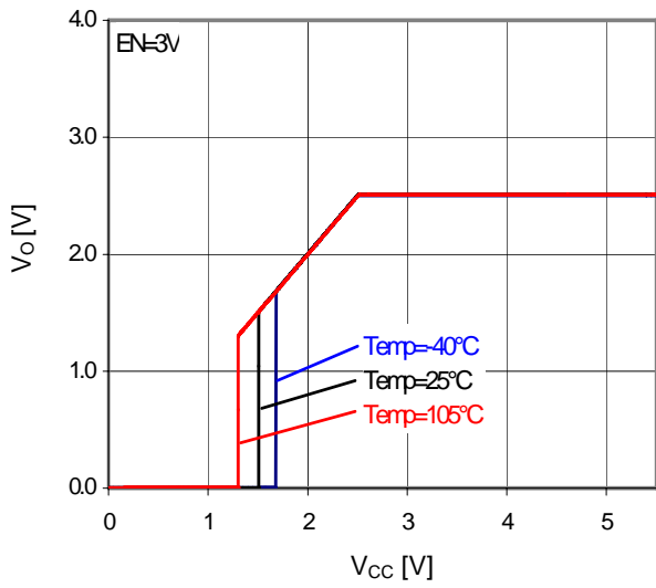
Fig.27 V_{cc}-V_o ( I_o=0mA )
