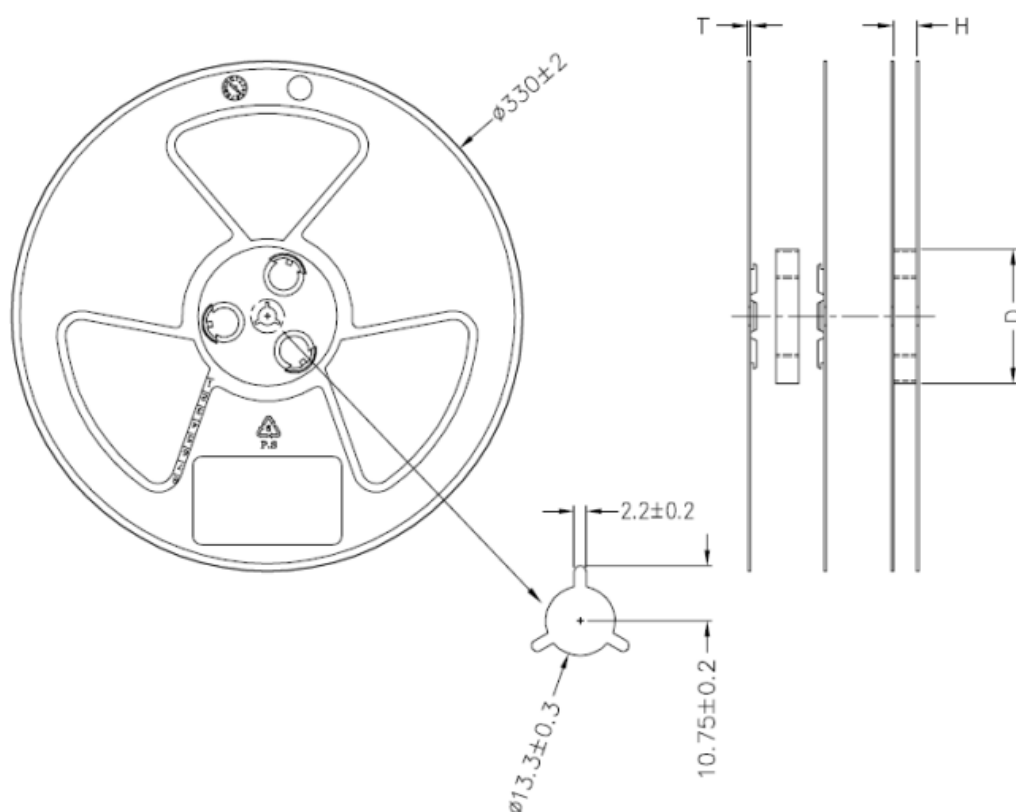
Fig. 5.1 Reel Dimension
