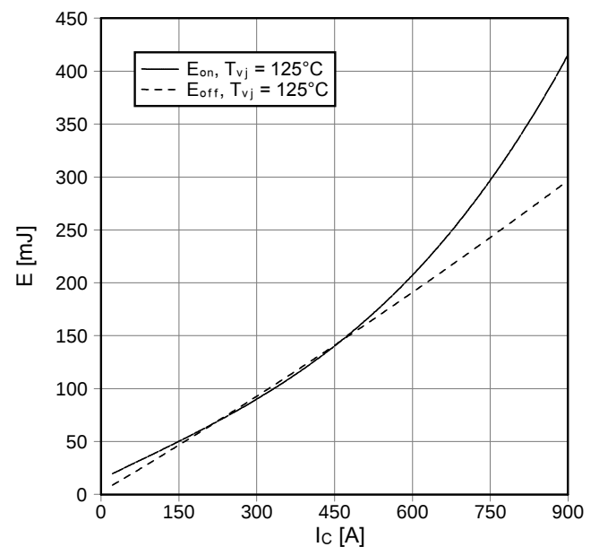
Schaltverluste IGBT-Wechselr. (typisch) switching losses IGBT-inverter (typical) E_{on} = f(I_C) , E_{off} = f(I_C) V_{GE} = \pm 15\text{ V} , R_{Gon} = 3,3\ \Omega , R_{Goff} = 3,3\ \Omega , V_{CE} = 900\text{ V}
