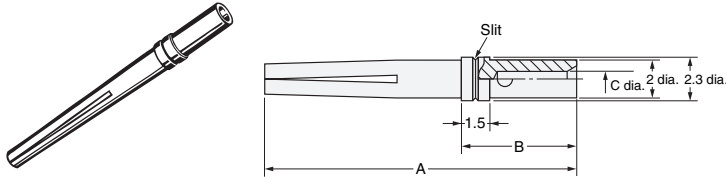
Dimensions
