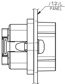
パネル後面取り付け REAR MOUNT TYPE
