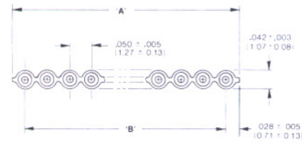
28 AWG SHOWN
