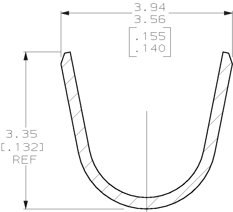
SECTION D-D SCALE 10:1
