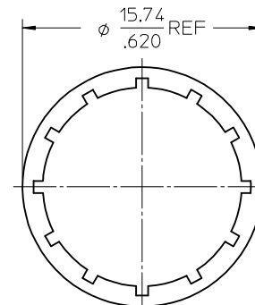
LOCKWASHER
