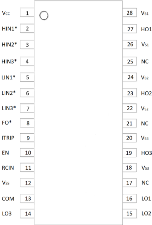
SO-28
