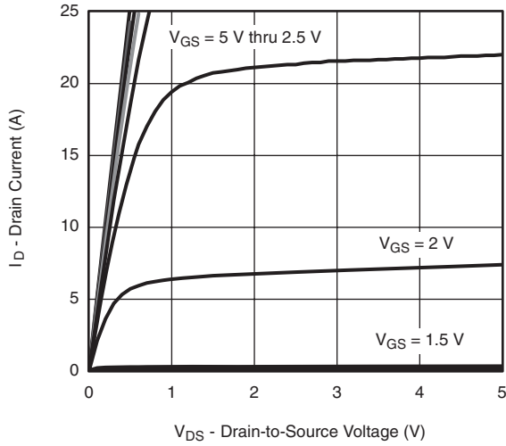
V_{GS} = 5\text{ V thru } 2.5\text{ V} V_{GS} = 2\text{ V} V_{GS} = 1.5\text{ V} Output Characteristics
