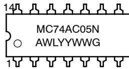
PDIP-14
