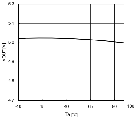
Fig.7 T_a - V_o ( I_o=0\text{mA} )
