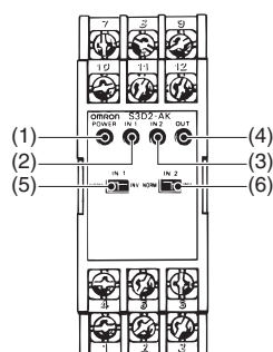
S3D2-AK/-AKD
