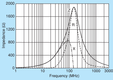
BLM21BD152SN1
