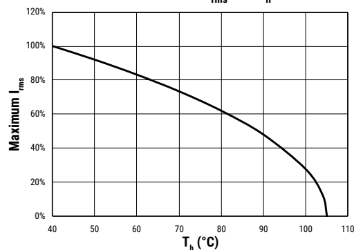
Maximum I_{rms} vs. T_h
